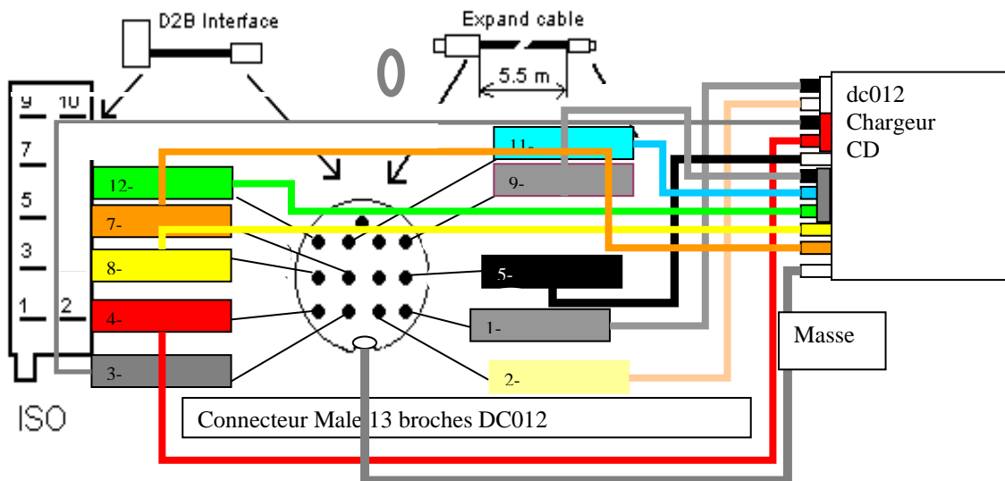
Couleur réelle des fils
